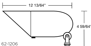
62-1206 62-1207 62-1208 PAR 30 Size
