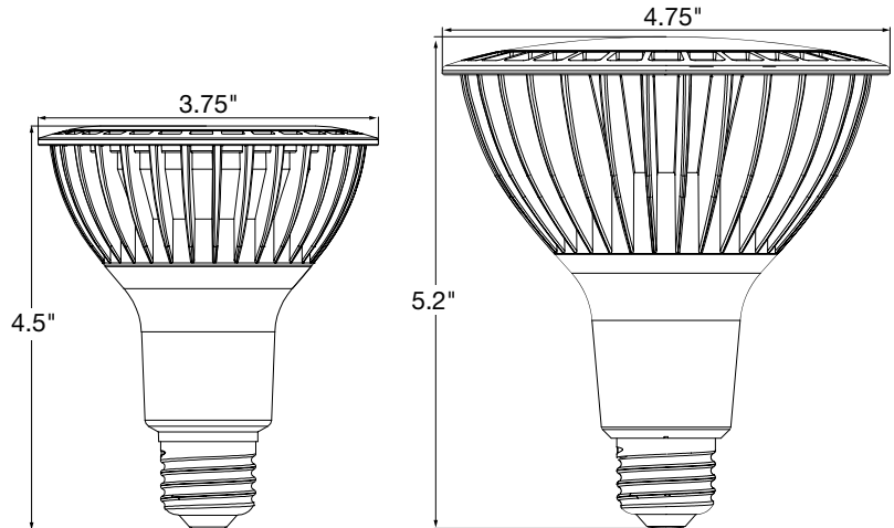
PAR 30
