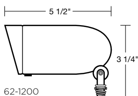
62-1200 62-1201 62-1202 PAR 16 Size
